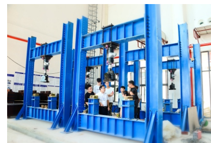
结构工程阵列加载试验系统
